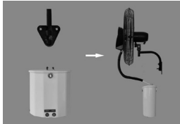
5. Su deposu ve buhar aparatı, su boru bağlantıları yapılmalı ve duvara montajlanmalı.
